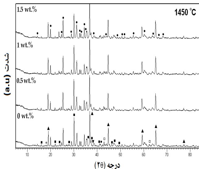
شکل (۱): تاثیر مقادیر مختلف نانوذرات اکسید کروم بر فازهای تشکیل شده در ترکیب سیمان پس از پخت ■:CA, ●:CA 2 , ▲:Spinel, ▽:Al 2 O 3 , □:MgO, ○:C 12 A 7
