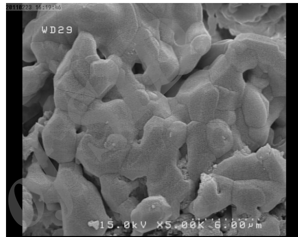
شکل (۴): تصویر میکروسکپ الکترونی مربوط به سطح شکست نمونه بدون نانوذرات اکسید کروم پس از پخت
