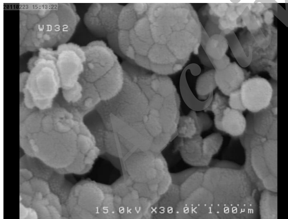
شکل (۶): تصویر میکروسکپ الکترونی مربوط به سطح شکست نمونه حاوی ۱/۵ درصد وزنی نانوذرات اکسید کروم پس از پخت
