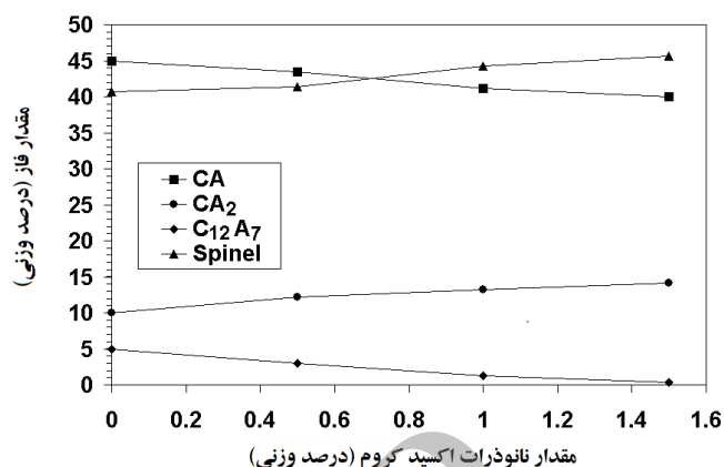
شکل (۴): تاثیر مقادیر مختلف نانوذرات اکسید کروم بر میزان فازهای تشکیل شده در ترکیب سیمان پس از پخت
