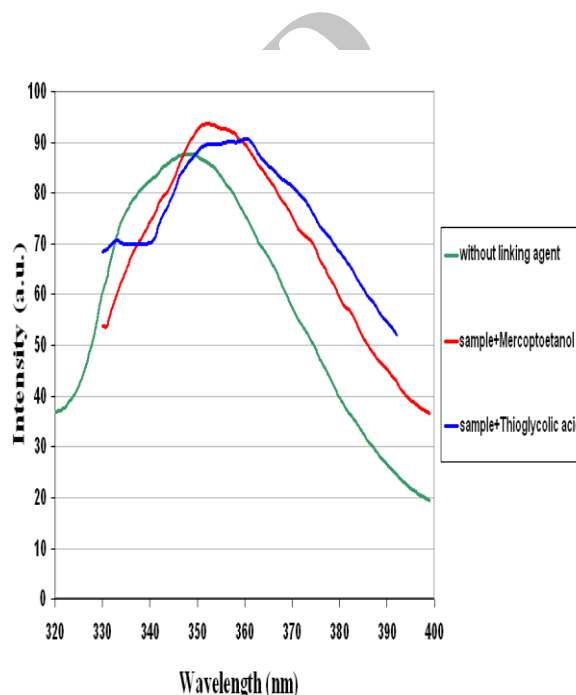
شکل (۶): طیف شدت گسیل نانوذرات ZnS:Mn بدون عامل اتصال و با مرکاپتواتانول و تیوگلیکولیک اسید
