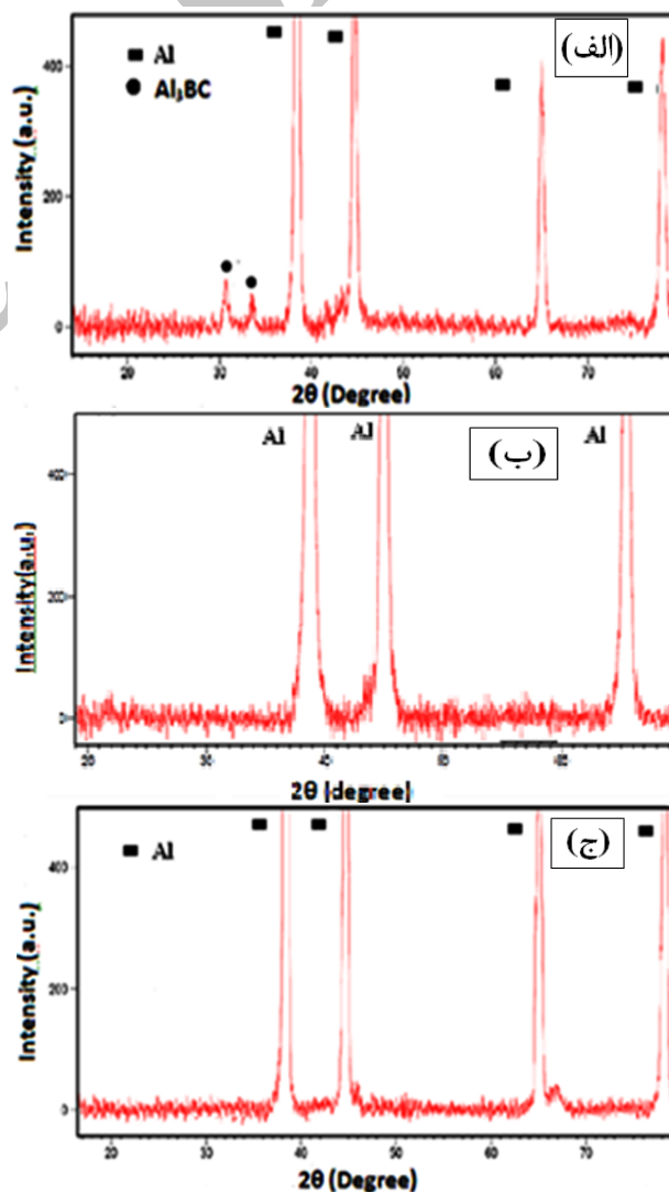
شکل (۴): الگوی پراش اشعه X نمونه های: الف) CA، ب) Mix و ج) MA
