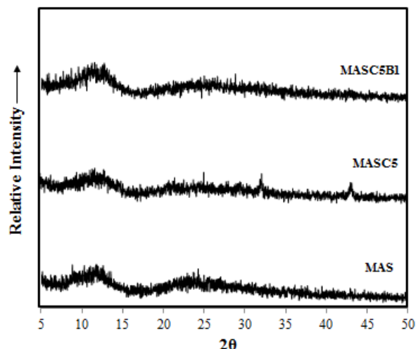
شکل (۳): الگوهای XRD ترکیبات آمورف حاصل از ژل کلسینه شده در 500^\circ\text{C}
