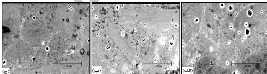
شکل (۸): تصاویر میکروسکوپ الکترونی فولاد ۳۲۱ محلول‌سازی شده در پتانسیل ۱ ولت و دمای: (الف) بدون حساس شدن، (ب) 600^{\circ}\text{C} ، (ج) 800^{\circ}\text{C}
