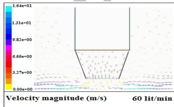
شکل (۱۱): بردارهای سرعت گاز در نرخ جریان ۶۰ Lit/min.
