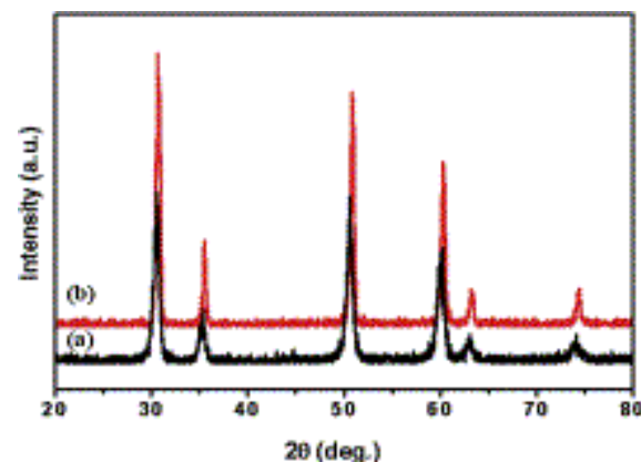
شکل (۳): الگوی پراش اشعه X پودر 8YSZ (a) نانو، 8YSZ میکرون (b).
