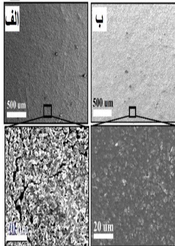
شکل (۷): تصاویر SEM از پوشش TBC پس از عملیات حرارتی در دمای 1000^{\circ}\text{C} (الف): میکروساختار و (ب): نانوساختار.
