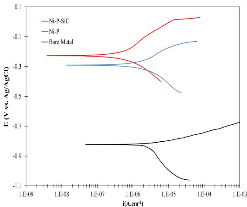
شکل (۶): منحنی های تافل پوشش های Ni-P، Ni-P-SiC و آلومینیوم بدون پوشش در محلول ۳٪ NaCl
