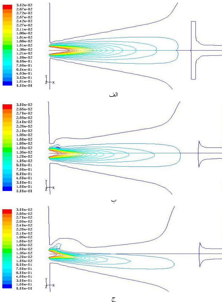
شکل (۶): توزیع سرعت برای افشانه پلازما: (الف): بدون گاز حامل، (ب): گاز حامل با سرعت ۵ m/s، (ج): گاز حامل با سرعت ۱۵ m/s
