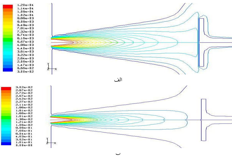
شکل (۲): توزیع دما برای افشانه پلاسما: (الف): بدون پروفایل، (ب): با پروفایل
