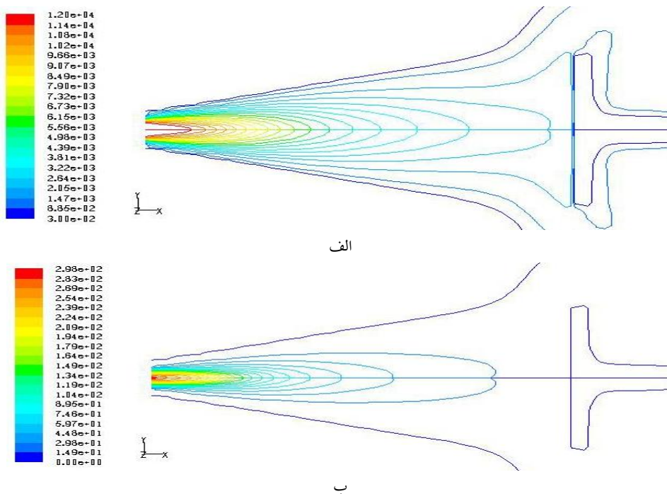
شکل (۳): توزیع سرعت برای افشانه پلاسما: (الف): بدون پروفایل، (ب): با پروفایل
