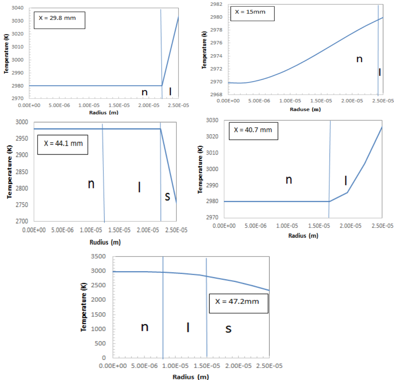
شکل (۱۴): تغییر فاز داخل یک ذره ( 50\mu m ) (بدون گاز حامل). خط عمودی سطح مشترک جامد-مایع با n نانو ساختار مواد، l ماده ذوب شده و s مواد انجماد نشان می دهد
