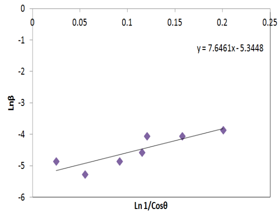
شکل (۵): نمودار کمترین مربعات خطا برای میکروکره‌های کامپوزیتی TiO_2/C
