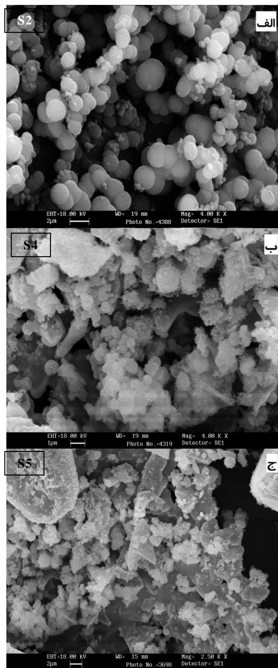
شکل (۳): اثر pH بر مورفولوژی و اندازه میکروکره های TiO_2/C : (الف): 0/8 ، (ب): 2 و (ج): 6
