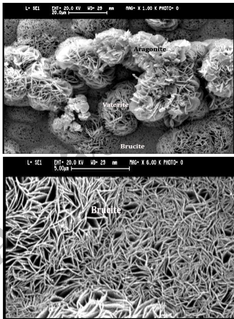
شکل (۶) تصویر تهیه شده توسط SEM رسوبات آهنی در آب دریای طبیعی در دمای ۲۵ درجه سانتی‌گراد بعد از ۴۸ ساعت
