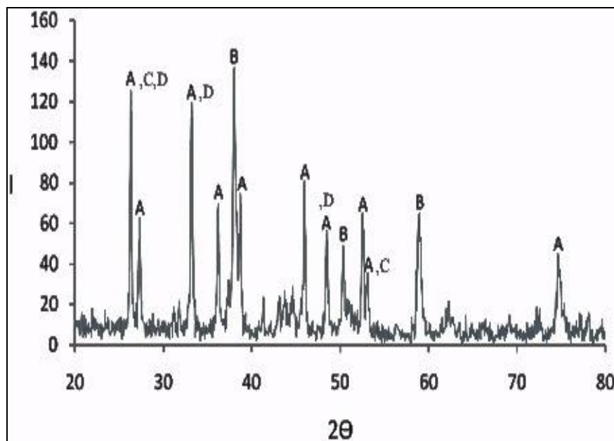
شکل (۴): نمودار آنالیز XRD مربوط به نمونه‌ها در دمای ۲۵ درجه سانتی‌گراد: A: (آراگونیت \text{CaCO}_3 )، B: (بوروکایت (\text{Mg}(\text{OH})_2) )، C: (کلسیت (\text{CaCO}_3) )، D: (واترایت (\text{CaCO}_3) )
