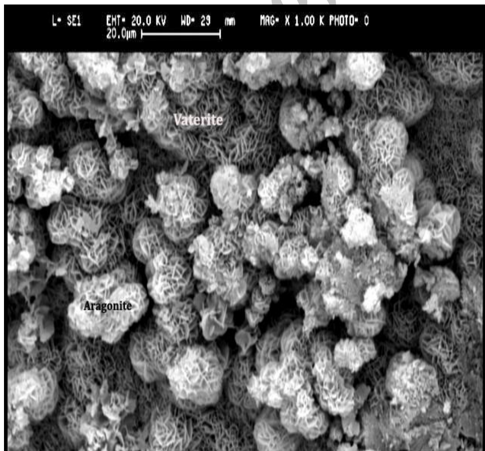
شکل (۳): تصویر تهیه شده توسط SEM رسوبات آهنی در آب دریای طبیعی در دمای ۲۵ درجه سانتی‌گراد بعد از ۲۴ ساعت
