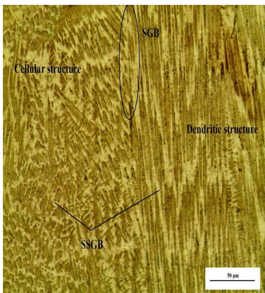
شکل (۱۰): ریزساختار سلولی-دندریتی فلز جوش ۳۱۰ در خط مرکزی جوش، نمایش حضور مرزدانه های فرعی انجماد و مرزدانه های انجمادی
