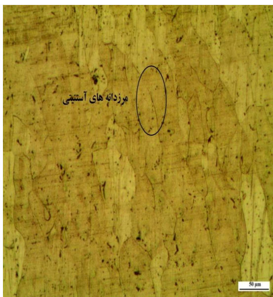
شکل (۸): ریزساختار فلز جوش اینکونل ۸۲
