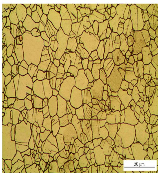
شکل (۴): ریز ساختار فلز پایه فولاد زنگ نزن آستنیتی ۳۱۰S (الف): حضور فريت دلتا در امتداد مرز دانه های آستنیتی، (ب): دو قلویی های ناشی از آنیل
