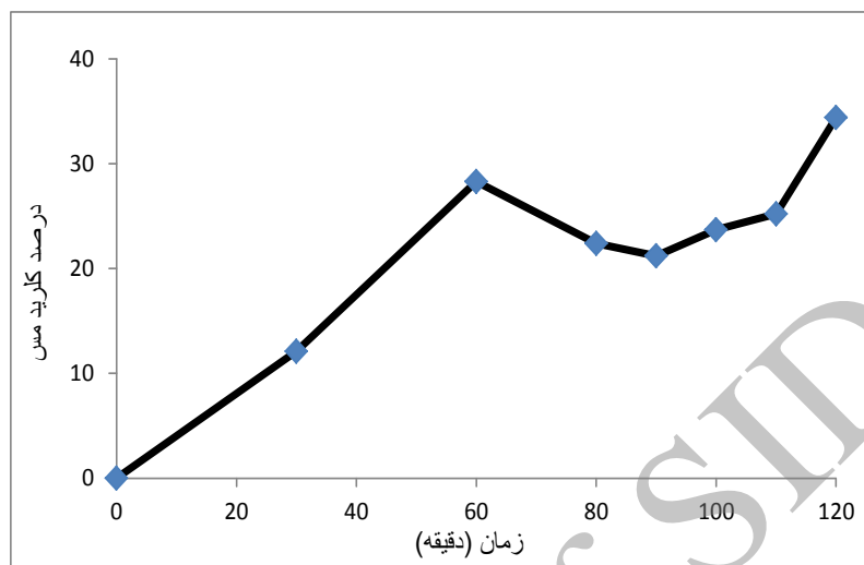
شکل (۴): درصد کلرید مس در زمان‌های مختلف کلراسیون و آسیاب کاری با نسبت گلوله به پودر ۱:۱۰
