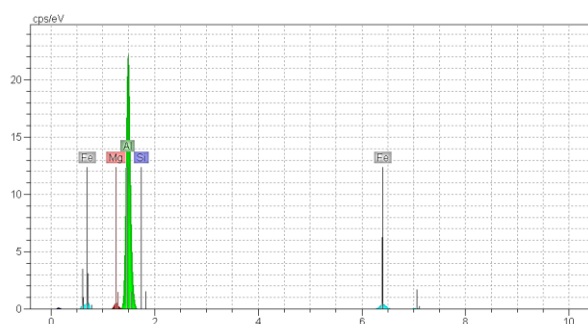
شکل (۱۴): آنالیز EDS از لایه ی بین فلزی اطراف تکه فولادی
