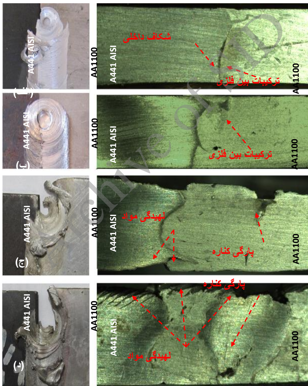
شکل (۱۴): پنجره ی اتصالی که در عمق نفوذ (الف): ۰/۱ میلیمتر، (ب): ۰/۲ میلیمتر، (ج): ۰/۴ میلیمتر و (د): ۰/۶ میلیمتر جوشکاری شد
