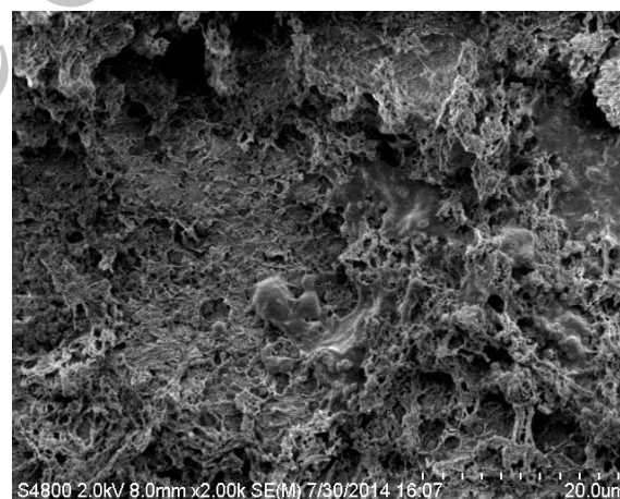
شکل (۷): تصویر میکروسکوپ الکترونی روبشی از سطح نانوکامپوزیت کایتوسن/مگنتیت بعد از هفت روز قرار گیری در محیط کشت
