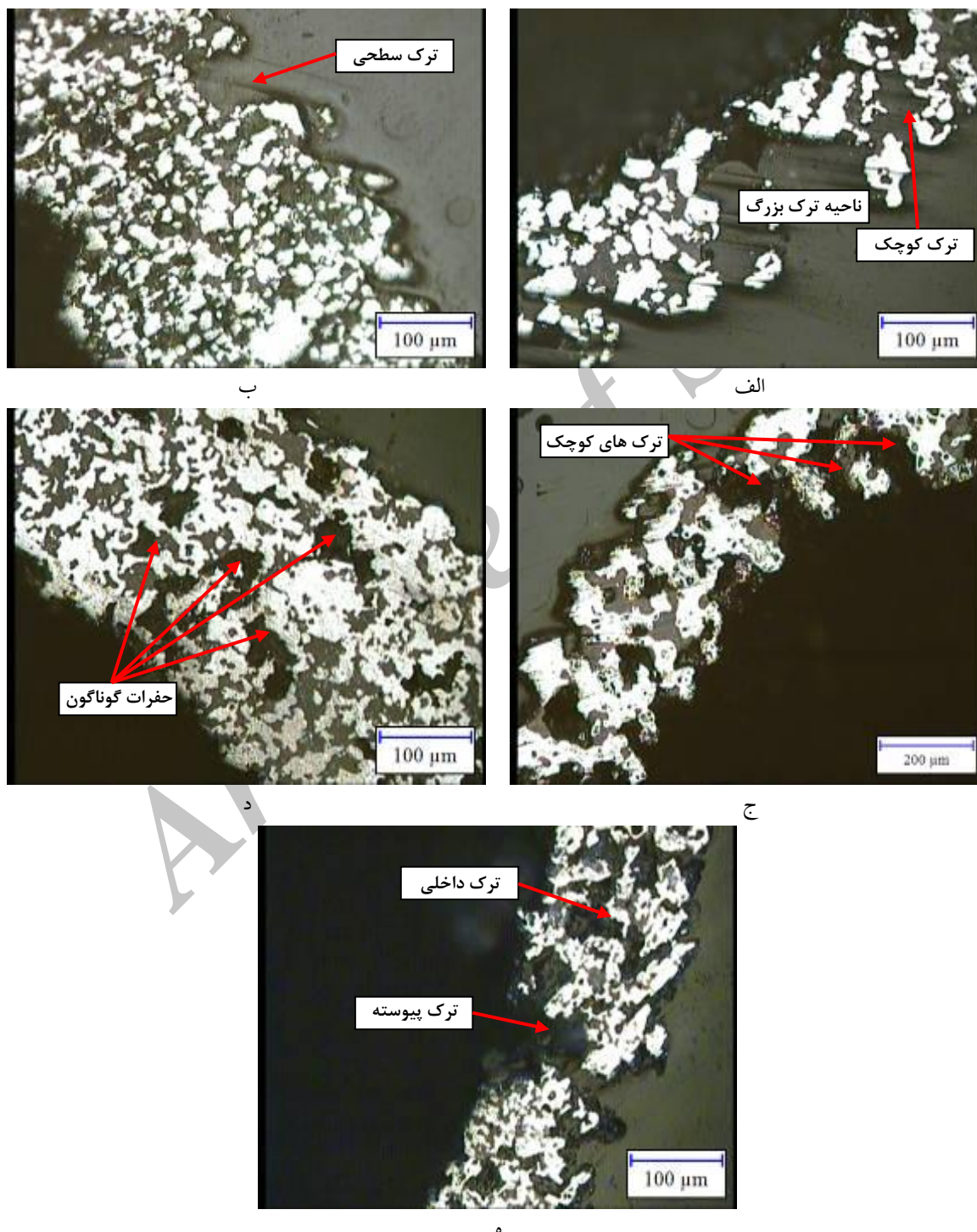
شکل (۴): نمایش ترک‌ها و حفرات ایجاد شده در پوسته گوی‌های فولادی: (الف): نمونه A، (ب): نمونه B، (ج): نمونه C، (د): نمونه D و (ه): نمونه E
