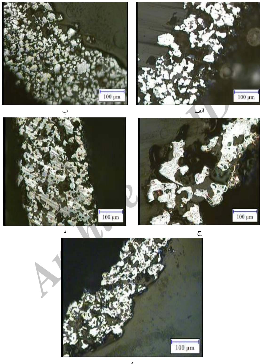
شکل (۲): تصاویر متالوگرافی از بخش مقطعی پوسته گوی‌های تولید شده: (الف): نمونه A، (ب): نمونه B، (ج): نمونه C، (د): نمونه D و (ه): نمونه E
