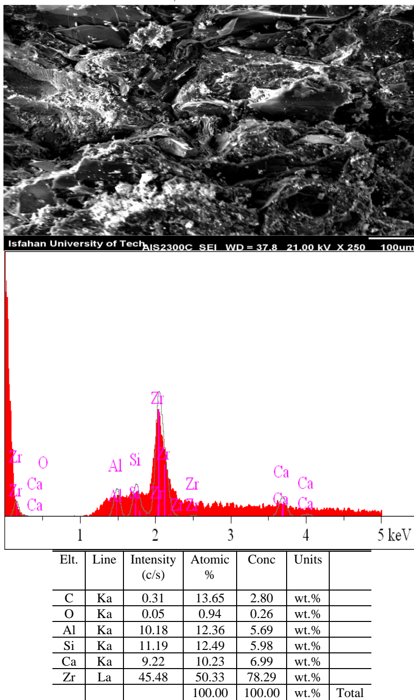
شکل (۴): تصویر تهیه شده توسط میکروسکوپ الکترونی روبشی و آنالیز EDS فازهای مشاهده شده در بدنه زیر کونیا گرافیت نازل سالم
