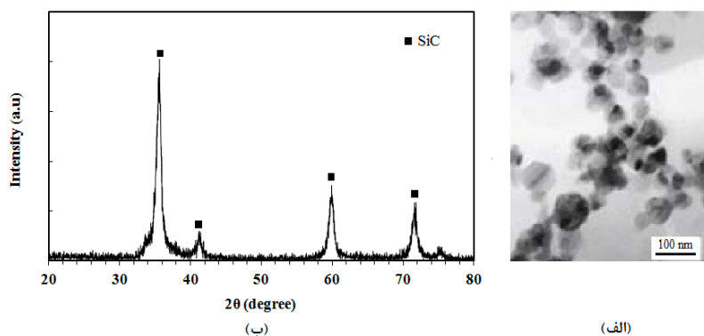
شکل (۱): (الف): تصویر TEM و (ب): الگوی XRD نانوذرات SiC
