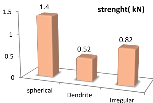
شکل (۷): نتایج آزمون ASTM1002 برای سه نوع پوشش کرومی، نامنظم و شاخواری
