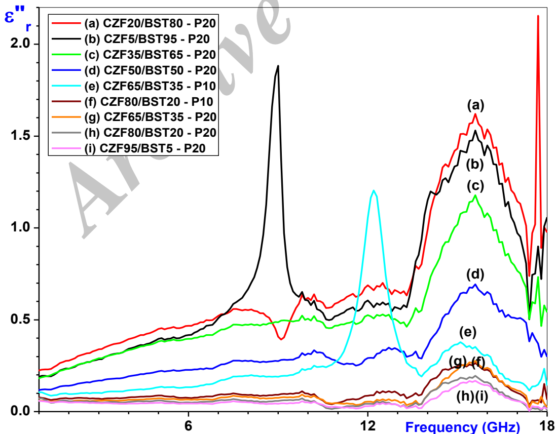
شکل (۴): تغییرات قسمت‌های موهومی گذردهی الکتریکی کامپوزیت‌های باریم استرانسیوم تیتانات/ فریت کبات-روی با درصد‌های پارافین متفاوت
