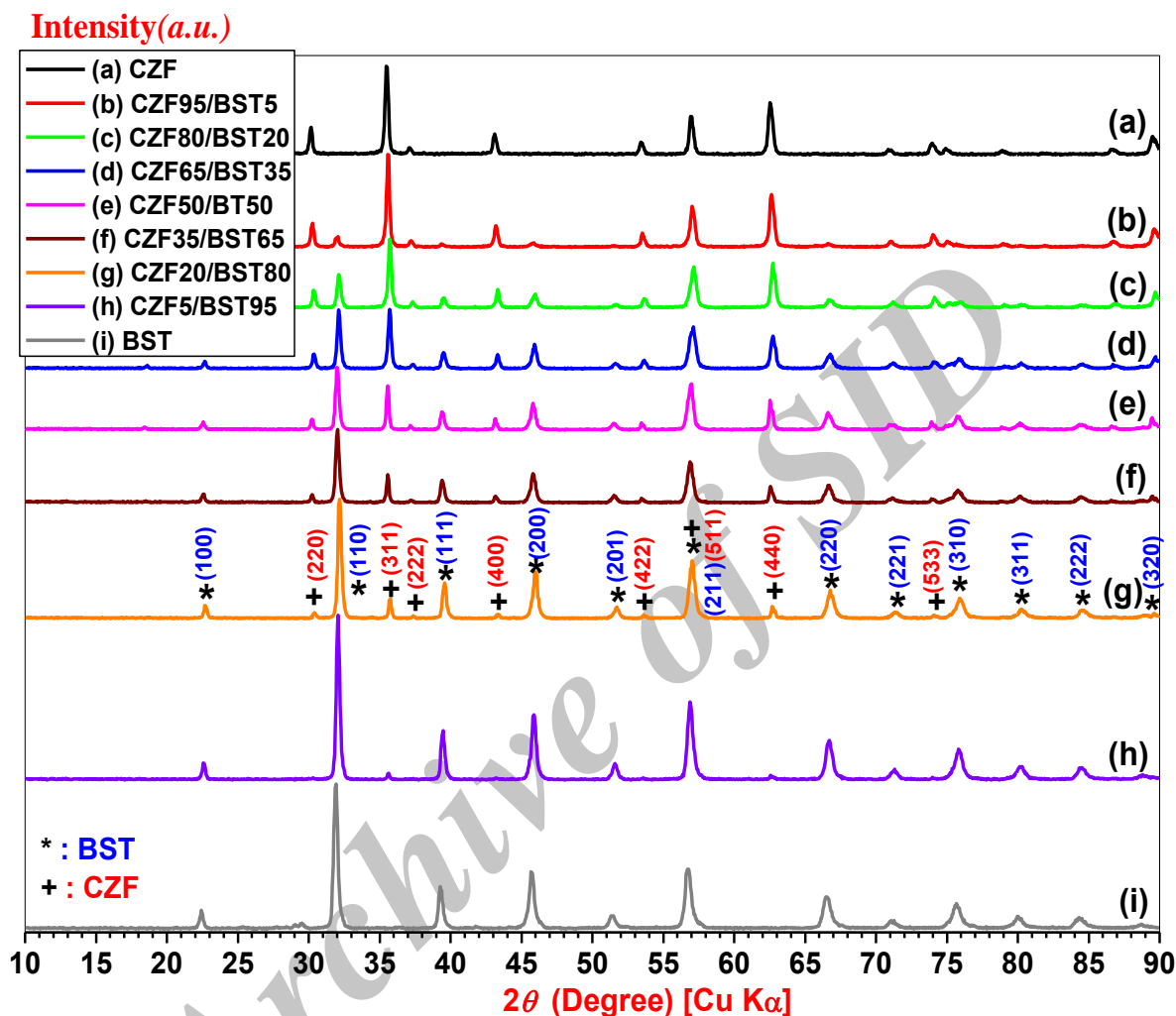
شکل (۲): طیف XRD مربوط به فریت کبات-روی، باریم استرانسیوم تیتانات و کامپوزیت‌های آن‌ها
