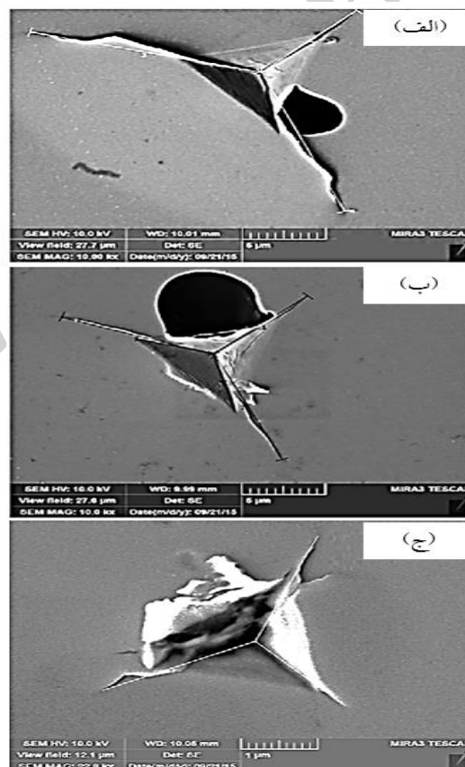
شكل (۲): تصاوير ميكروسكوپي الكتروني از سطح نمونه‌هاي نيتري تانتالوم تحت بارگذاري با نيروي بالا: (الف): TaN_{10} ، (ب): TaN_{15} و (ج): TaN_{25}
