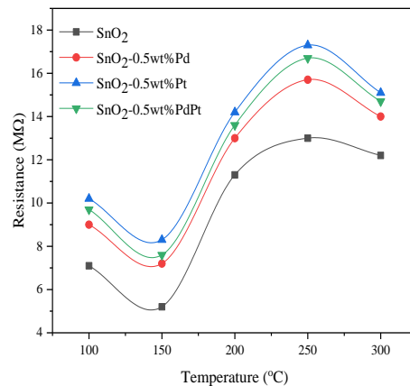
شکل (۷): تغییرات مقاومت بر حسب دما برای SnO 2 و هیبریدهای آن با مختلف Pt و Pd
