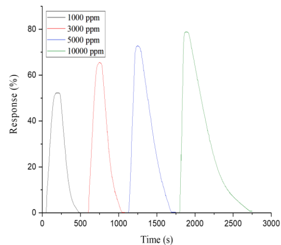
شکل (۱۰): نمودار پاسخ بر حسب غلظت متان برای حسگر هیبریدی \text{SnO}_2\text{-0.5wt\%PdPt} در دمای ۲۰۰ درجه سانتیگراد
