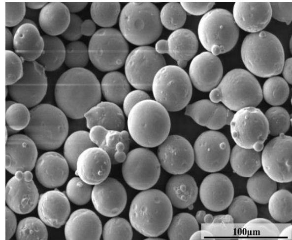
شکل (۱): مورفولوژی پودر تغذیه‌ی NiCrBSi
