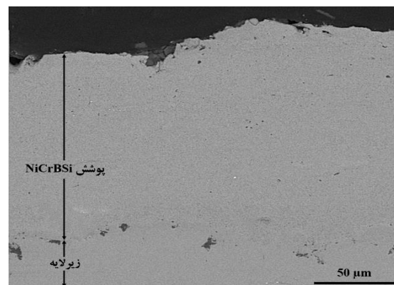
شکل (۹): تصویر SEM از سطح مقطع پوشش گداخت شده در دمای ۱۰۰۰°C و زمان ۵ دقیقه
