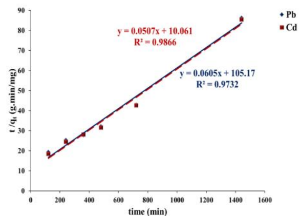
شکل (۹): سینتیک شبه مرتبه دوم در جذب کاتیون‌های سرب و کادمیم توسط جاذب نانو کامپوزیت پلی آکریل آمید-پلی استایرن/بنتونیت
