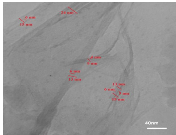
شکل (۵): تصویر TEM نانوکامپوزیت پلی‌آکریل‌آمید-پلی استایرن/بنتونیت
