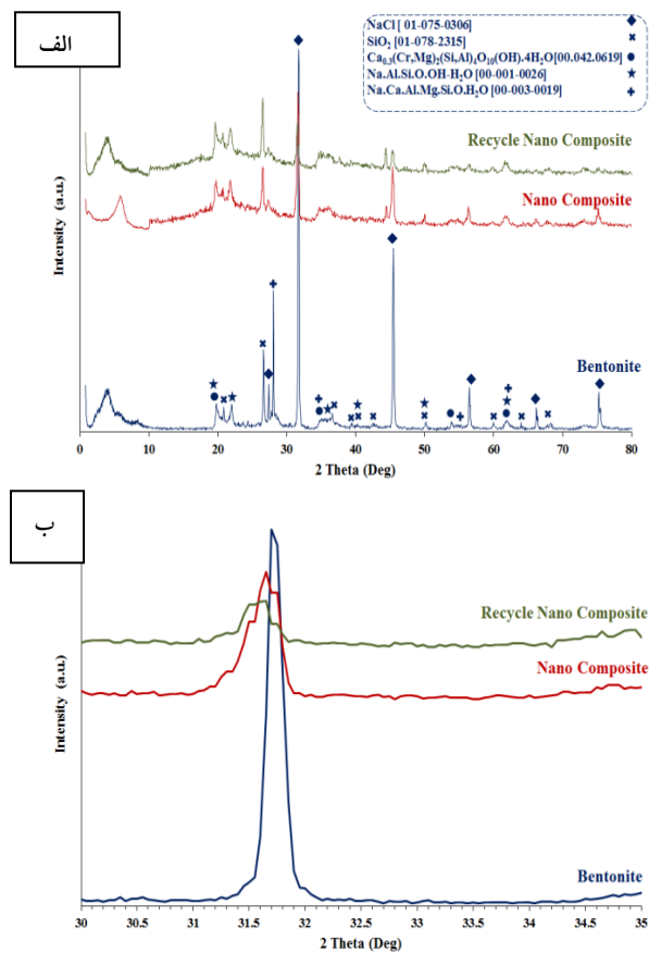
شکل (۱): (الف): تصویر پراش پرتو ایکس بنتونیت، نانو کامپوزیت پلی آکریل آمید- پلی استایرن/بنتونیت و نانو کامپوزیت پلی آکریل آمید- پلی استایرن/بنتونیت بازایی شده در 2\theta=0-80 و (ب): بنتونیت، نانو کامپوزیت پلی آکریل آمید- پلی استایرن/بنتونیت و نانو کامپوزیت پلی آکریل آمید- پلی استایرن/بنتونیت بازایی شده در 2\theta=30-35
