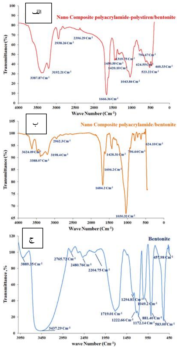
شکل (۲): طیف‌های مادون قرمز: (الف): بنتونیت، (ب): نانو کامپوزیت پلی آکریل آمید- پلی استایرن/بنتونیت و (ج): نانو کامپوزیت پلی آکریل آمید- بنتونیت
