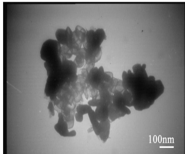
شکل (۱): تصویر میکروسکوپ الکترونی عبوری از نانوذرات دی سولفید تنگستن تولید شده
