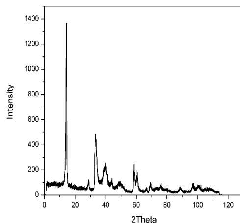
شکل (۲): نتایج آنالیز XRD دی سولفید تنگستن سنتز شده
