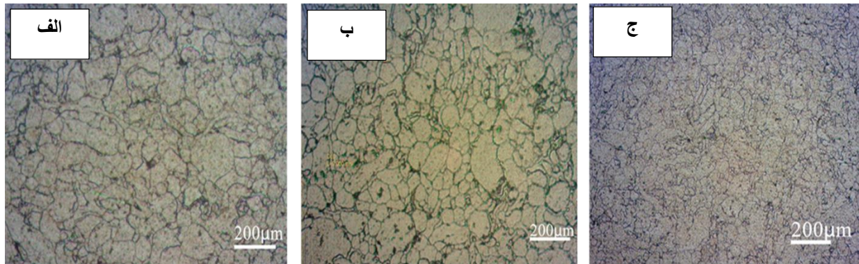
شکل (۳): تصویر میکروسکوپ نوری از سطح: (الف): نمونه خالص آلومینیوم، (ب): نمونه Al-2% WS 2 و (ج): نمونه Al-8% WS 2
