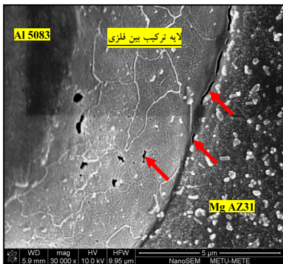
شکل (۶): حفرات کرکندال و رسوبات متعدد در فصل مشترک جوش نفوذی انجام شده در دمای اتصال دهی ۴۴۰ °C و در زمان اتصال دهی min ۶۰
