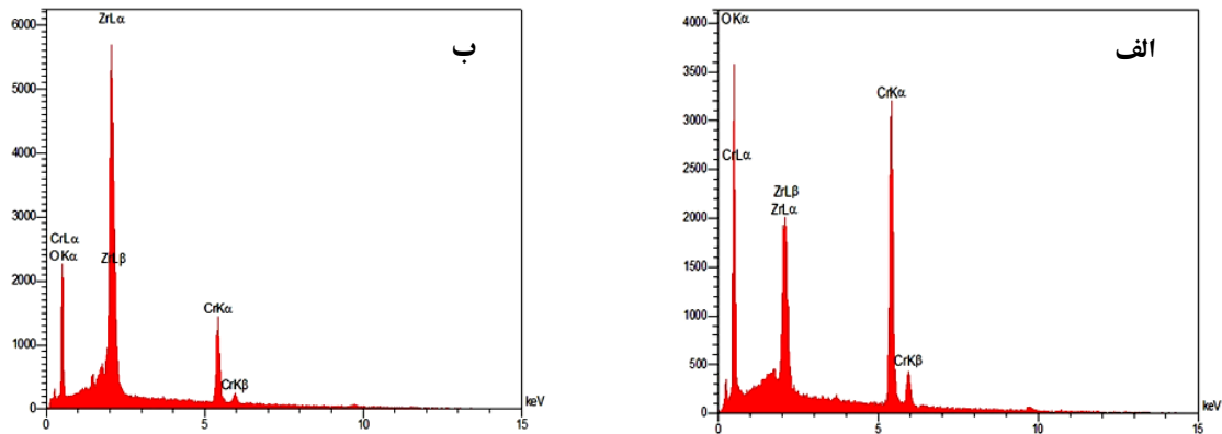
شکل (۸) - آنالیز عنصری از فازهای مختلف در پوشش CZ: الف) \text{Cr}_2\text{O}_3 (منطقه تیره رنگ در شکل ۷ (و)) ب) YSZ (نقاط روشن در شکل ۷ (و)).
