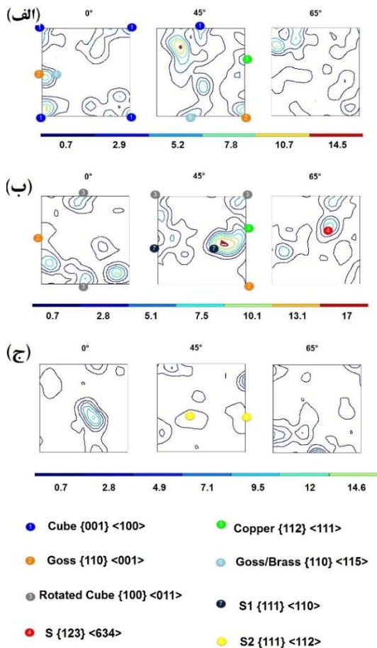
شکل (۴): مقاطع \phi=0^\circ ، 45^\circ و 65^\circ از توابع توزیع جهت گیری برای نمونه‌های الف (S-A، ب) S-O و ج) S-W.
