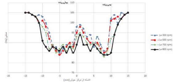
شکل (۱۷): تغییرات پروفیل سختی ورق ۵ میلی متری کار سرد شده بر اثر تغییرات سرعت دورانی
