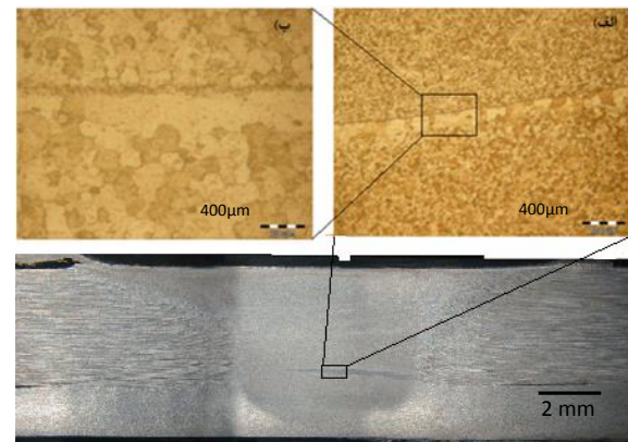
شکل (۸): عیب نقص پیوندی ۵۰۰ rpm، الف) درشت ساختار و ب) ریزساختار.
