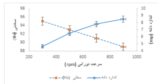
شکل (۱۰): تغییرات سختی و اندازه دانه مرکز جوش بر اثر تغییر سرعت دورانی در سرعت پیشروی ثابت (۴۵ mm/min).
