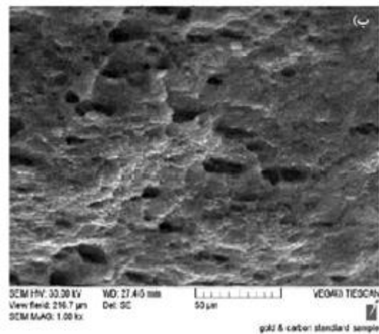
شکل (۱۹): تصویر میکروسکوپ الکترون روبشی از سطح شکست آزمون کشش نمونه جوشکاری شده با ۷۰۰ rpm (الف) بزرگنمایی ۲۰۰X و (ب) بزرگنمایی ۱۰۰۰X.
