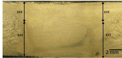
شکل (۱۳): ضخامت مؤثر ورق (EST) در دو ورق برای نمونه ۹۰۰ rpm
