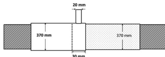
شکل (۳): شماتیک نمونه جوشکاری شده.
