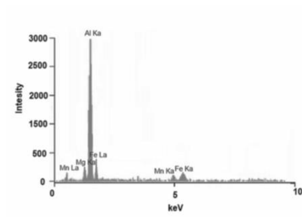
شکل (۱۲): آنالیز EDX ذرات مشاهده شده در شکل (۱۱)
