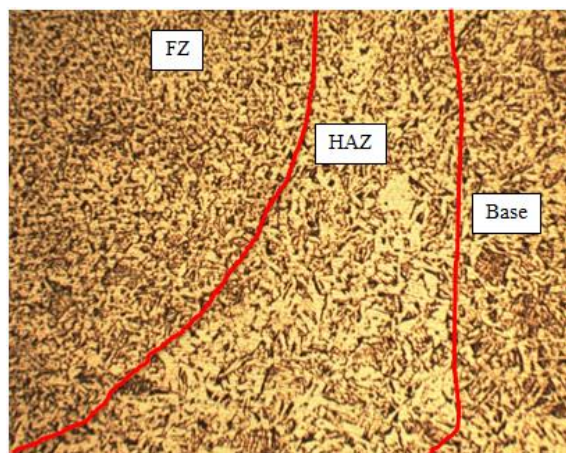
شکل (۱۵): ریز ساختار ناحیه جوش کاری شده با حضور ۰/۵ گرم نانو ذرات
