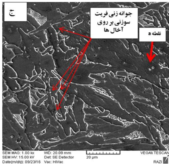
شکل (۱۰): تصاویر SEM: الف) دانه بندی فلز پایه، ب) ساختار فلز جوش بدون نانو ذرات و ج) ساختار فلز جوش با نانو ذرات وجود آخال‌های ریز به عنوان مراکز جوانه زنی فریت سوزنی
