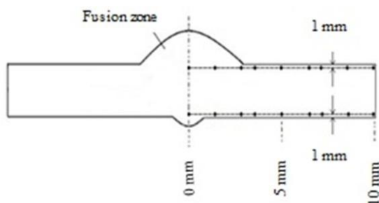
شکل (۴): نقاط نمونه مورد بررسی برای میکرو سختی
