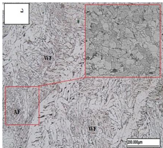
شکل (۹): مقایسه ساختار فلز جوش با بزرگنمایی مختلف: الف، ب، نمونه بدون ذرات نانو ذرات. ج، د، نمونه با ذرات نانو. AF: فريت سوزنی، PF: فريت چند وجهی و WF: ویدمن اشتاتن
