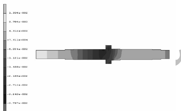
شکل (۶): مقدار جابه‌جایی در راستای محور Y که ماکزیمم ۰/۰۱ میلی‌متر
