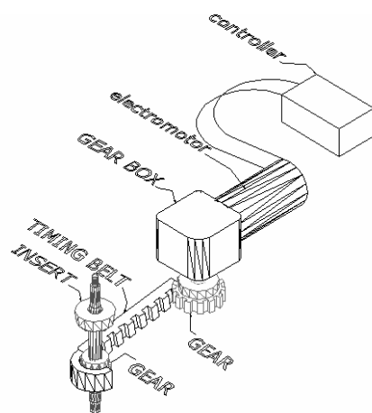
شکل (۲): نمای شماتیک از مکانیزم تامین نیرو
