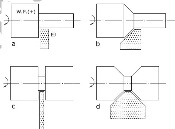
شکل (۹): استفاده از جت الکتروشیمیایی با اشکال هندسی به شکل پروفیل قطعه کار در تراشکاری با جت الکتروشیمیایی
