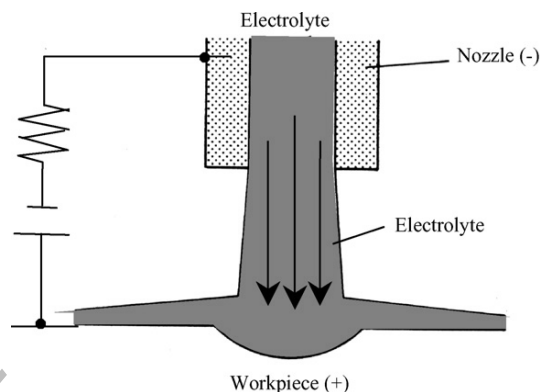
شکل (۳): استفاده از جت الکتروشیمیایی در ماشینکاری الکتروشیمیایی [۹]
