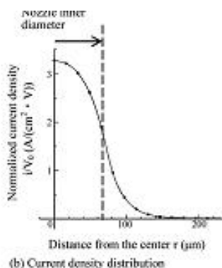
شکل (۴): (a) توزیع پتانسیل الکتریکی و (b) توزیع دانسیته جریان در جت الکتروشیمیایی [۱۰]
