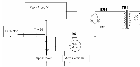
شکل (۶): شماتیک مدار کنترلی دستگاه ساخته شده
