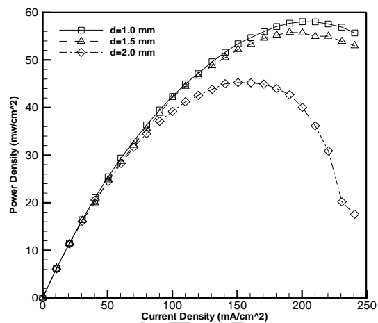
شکل (۸): (الف) نمودار تغییرات دانسیته توان-دانسیته جریان (ب) نمودار تغییرات ولتاژ- دانسیته جریان (غلظت محلول متانول ۱ مولار)
