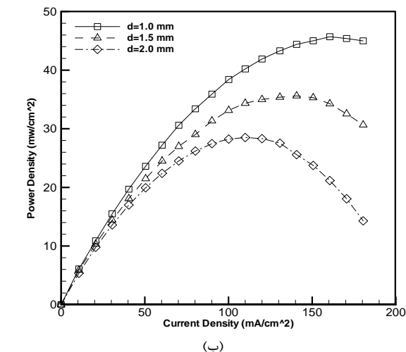
شکل (۱۰): (الف) نمودار تغییرات دانسیته توان-دانسیته جریان (ب) نمودار تغییرات ولتاژ- دانسیته جریان (غلظت محلول متانول ۱/۵ مولار)
