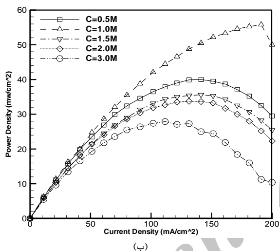
شکل (۴): (الف) نمودار تغییرات ولتاژ-دانشسته جریان (ب) نمودار تغییرات دانشسته توان-دانشسته جریان (عمق کانال ۱/۵ میلی‌متر)
