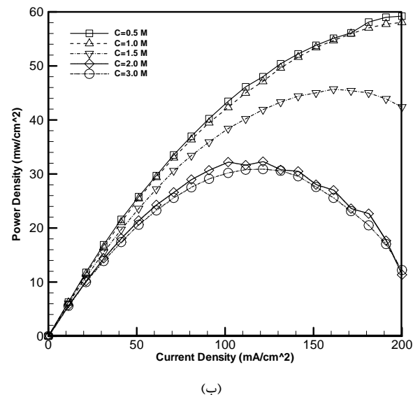
شکل (۳): (الف) نمودار تغییرات ولتاژ-دانشسته جریان (ب) نمودار تغییرات دانشسته توان - دانشسته جریان (عمق کانال ۱ میلی‌متر)
