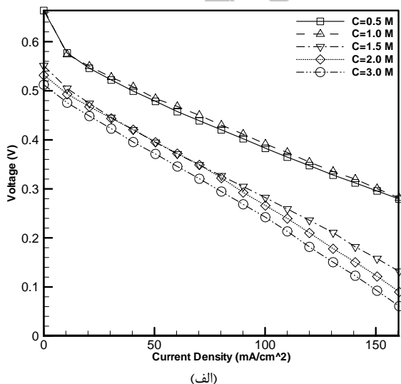
شکل (۴): (الف) نمودار تغییرات ولتاژ-دانشسته جریان (ب) نمودار تغییرات دانشسته توان-دانشسته جریان (عمق کانال ۱/۵ میلی‌متر)
