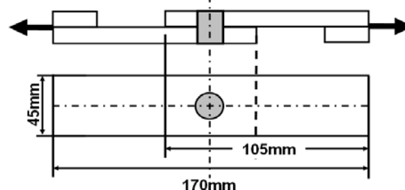
شکل (۲): ابعاد تست کشش-برش
