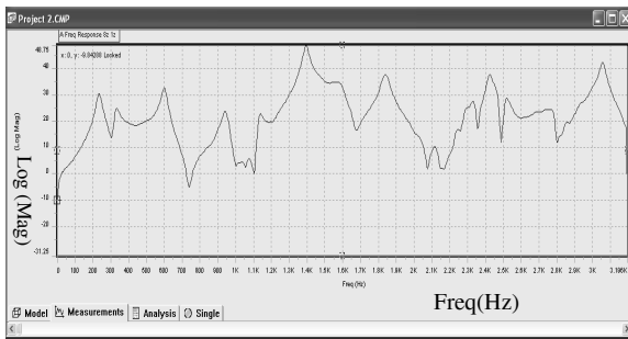
شکل ۴. نمودار دامنه فاز تابع پاسخ فرکانسی H18 (تحریک در نقطه ۸ و اندازه‌گیری در ۱)
