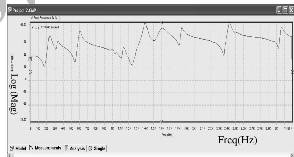
شکل ۳. نمودار دامنه فاز تابع پاسخ فرکانسی H11 (تحریک در نقطه ۱ و اندازه‌گیری در نقطه ۱)
