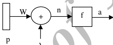
شکل ۱ ساختار نرون تک‌ورودی
