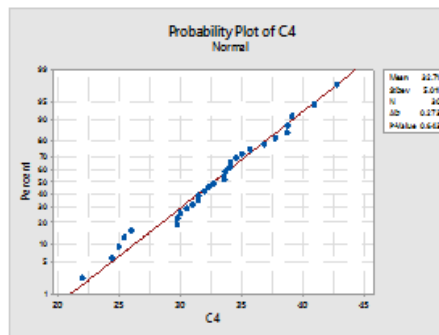
شکل ۵ نمودار نرمال بودن مشاهدات سیستم واقعی
