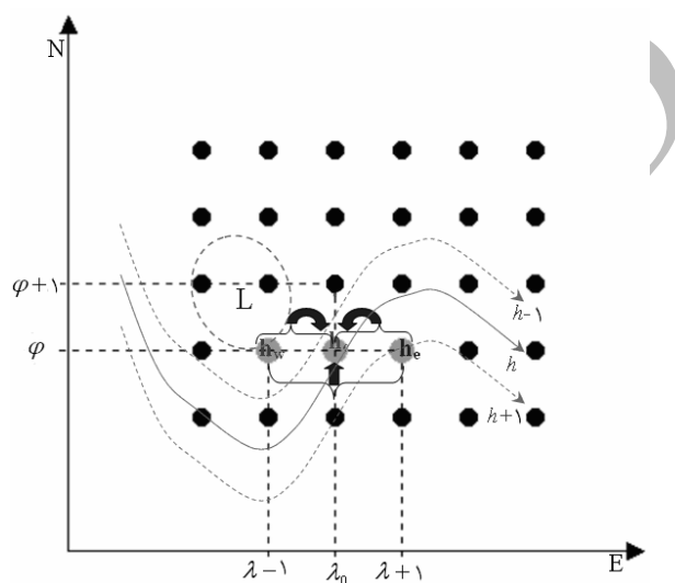
شکل ۱ فرایند محاسبه پیشرو در مدل PSP در الگوی یک سیستم کم‌ارتفاع بسته در سطح ۰۰۰ هکتوپاسکال در ماتریس محاسباتی
