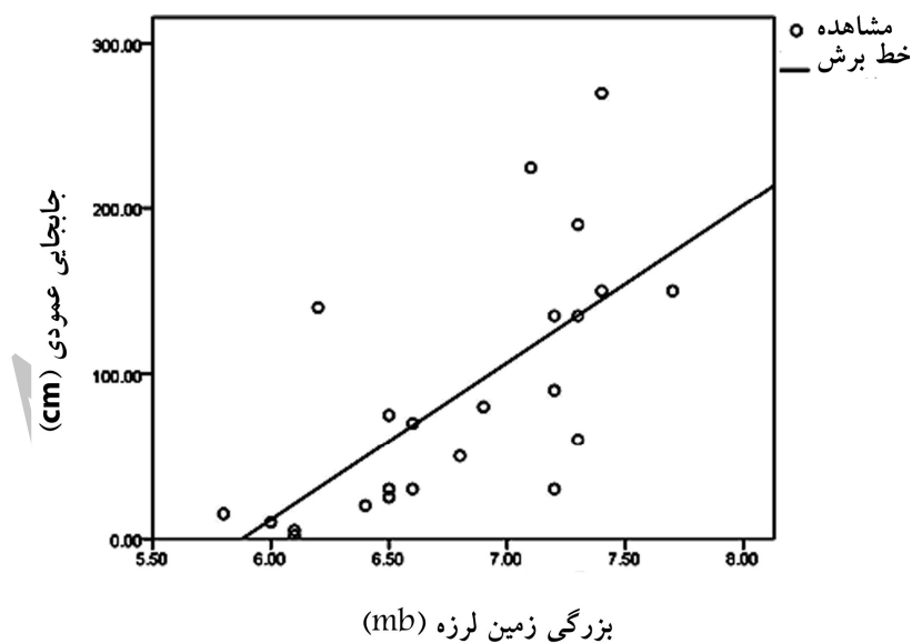
شکل ۷ ارتباط بين بزرگاي زمين‌لرزه و حرکت عمودي زمين
