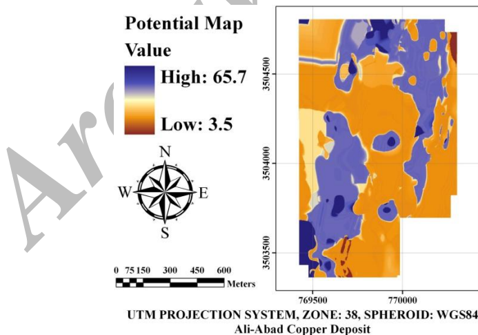
شکل ۶ نقشه پتانسیل معدنی زمین‌شناسی با استفاده از سیستم استنتاج فازی ژنتیک
