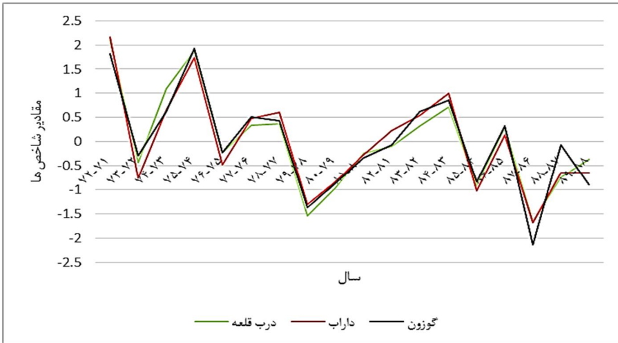
شکل 2 نمودار شاخص SPI در ایستگاه‌های داراب، درب‌قلعه و گوزون از سال آبی 1371-1389
