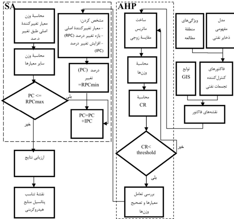
شکل 2 فلوچارت روش AHP و SA برای تهیه نقشه تناسب پتانسیل منابع هیدروکربنی
