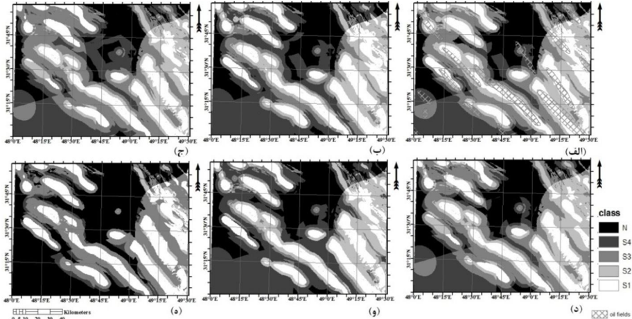
شکل 5 الف- نقشه تناسب حاصل از اجرای پایه؛ ب- نقشه تناسب با معیار تغییرکننده اصلی شاخص TOC با تغییر وزن 2%؛ ج- نقشه تناسب با معیار تغییرکننده اصلی شاخص S_1+S_2 با تغییر وزن 2%؛ د- نقشه تناسب با معیار تغییرکننده اصلی شاخص T_{max} با تغییر وزن 4%؛ ه- نقشه تناسب با معیار تغییرکننده اصلی مجاورت با محور طاق‌دیس‌ها با تغییر وزن 2%؛ و- نقشه تناسب با معیار تغییرکننده اصلی وجود مناطق دارای آنومالی ثقل بوگه بالا یا مجاورت با آنها با تغییر وزن 2%
