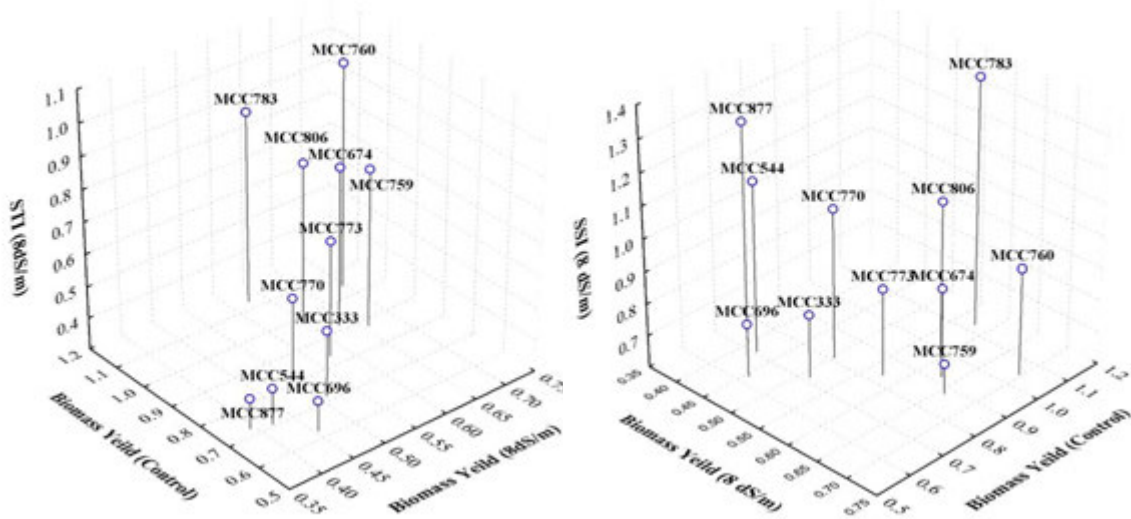
شکل ۲- نمودار سه‌بعدی تغییرات میانگین تولید ماده خشک در تیمار شاهد، میانگین تولید ماده خشک در تیمار 8dSm^{-1} با مقدار STI8 و SSI8 در نخود
