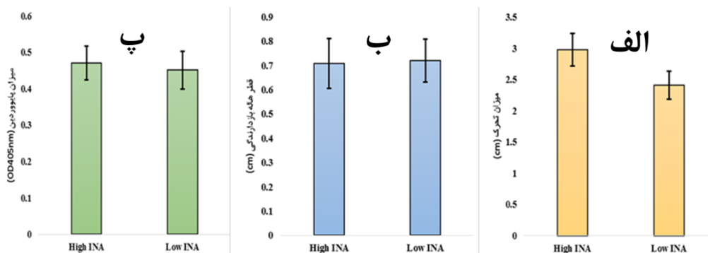
شکل ۳. مقایسه سه فاکتور مؤثر در بیماری‌زایی میان دو قدرت هسته یخ‌زدگی. (الف) میزان تحرک، (ب) میزان حساسیت به H_2O_2 ، (پ) میزان تولید سیدروفور پایووردین
