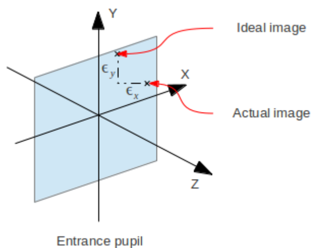
شکل ۴. پرده تصویر و مختصه پرتویی ابیراهی یافته نسبت به شرایط ایده آل
