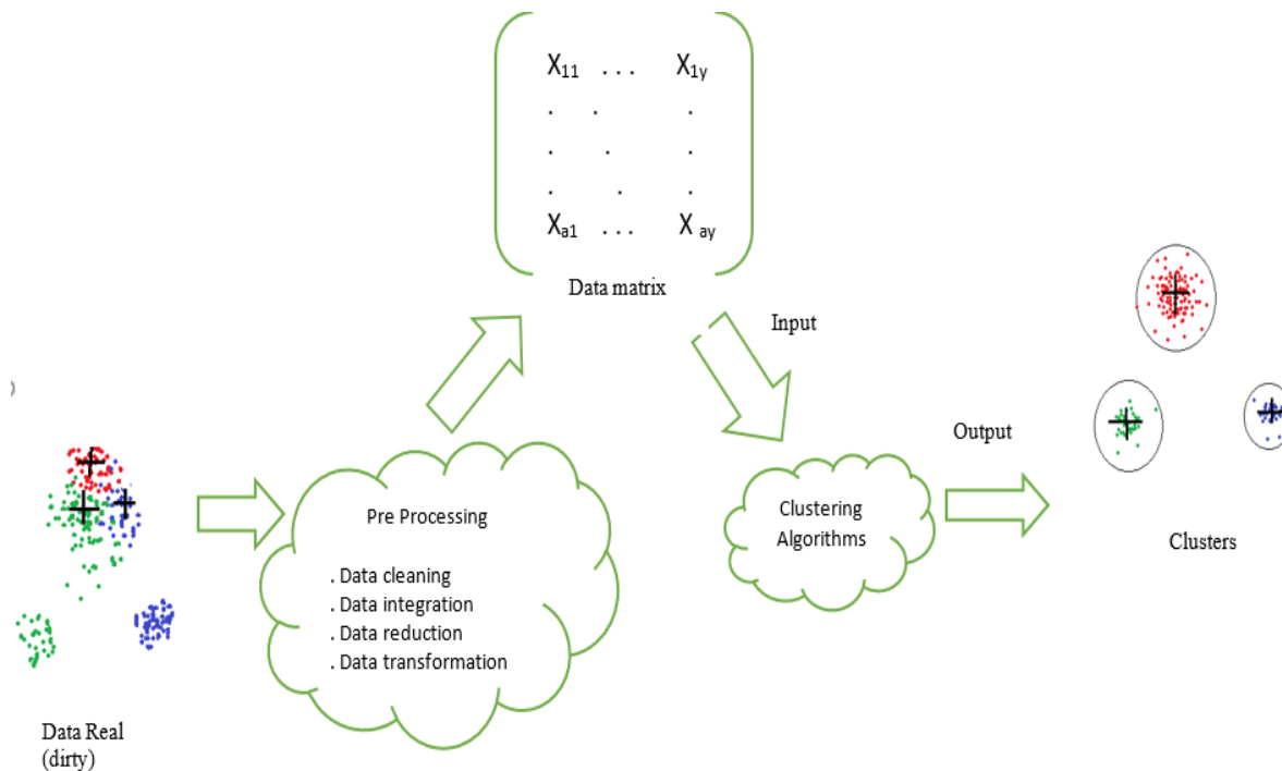
شکل ۲- فرایند خوشه‌بندی [۶]
