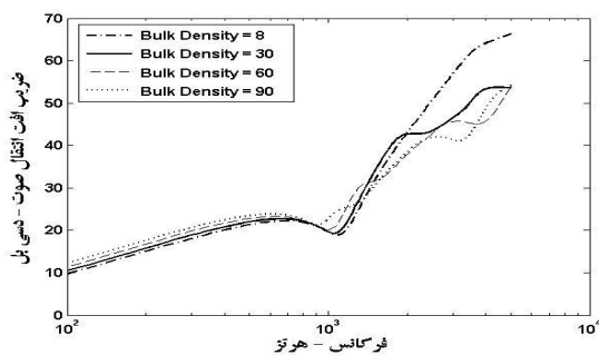
شکل (۱۵) اثر چگالی بالک بر TL در حالت (B-B).
