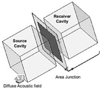
شکل (۵) مدل SEA سازه پنل دوجداره با لایه متخلخل میانی به همراه جریان توان بین هر سه زیرسیستم.
