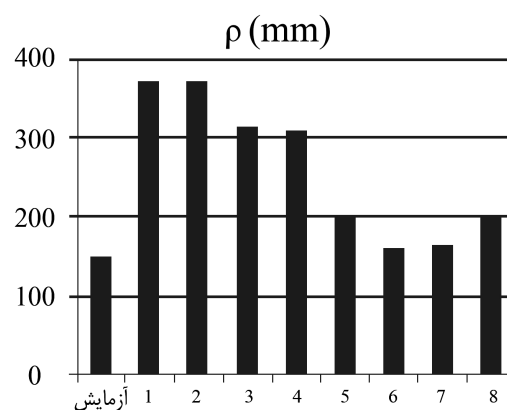
شکل (۷) مقادیر شعاع انحنا دیواره جانبی برای حالات مختلف شبیه‌سازی وقتی ضریب اصطکاک ۰/۱، نیروی ورقگیر ۲۰ kN، استحکام تسلیم ورق ۳۶۵ MPa و ضخامت ورق ۱ mm است.
