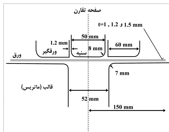
شکل (۳) نمایش شماتیک هندسه قالب.
