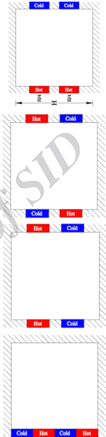
شکل (۱) چهار حالت در در نظر گرفته شده برای المان‌های حرارتی
