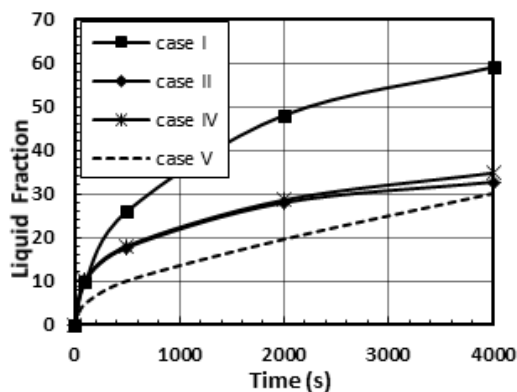
شکل (۱۴) تغییرات کسر مایع در چیدمان‌های مختلف برای بکارگیری صفر درصد نانو ذره اکسید آلومینیوم
