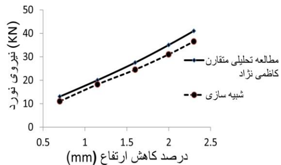
شکل (۱۰) تأثیر درصد کاهش ارتفاع بر نیروی نورد و مقایسه با حالت نورد
